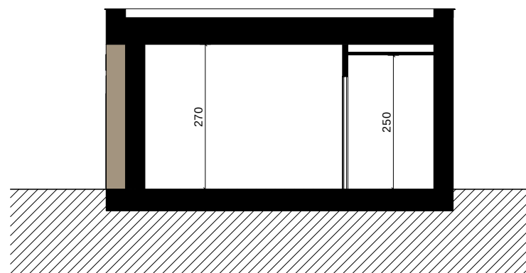
Sezione BB
